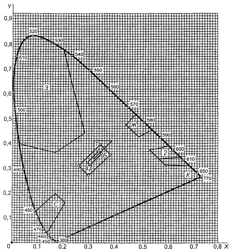
Колориметрические и фотометрические характеристики сигнальных и контрастных цветов элементов ФЭС, знаков безопасности и сигнальной разметки
