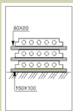
Плиты перекрытия
